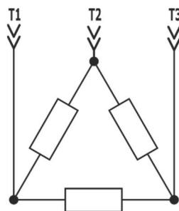
Dreieckschaltung
